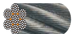
âme métal - 7 x 19 fils
