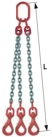
3 crochets à touret à verrouillage automatique
