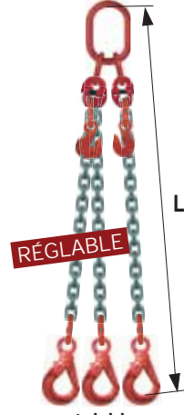
réglable 3 crochets à verrouillage automatique
